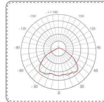
DISTRIBUCIÓN DE LA INTENSIDAD LUMÍNICA
