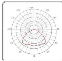
DISTRIBUCIÓN DE LA INTENSIDAD LUMÍNICA
